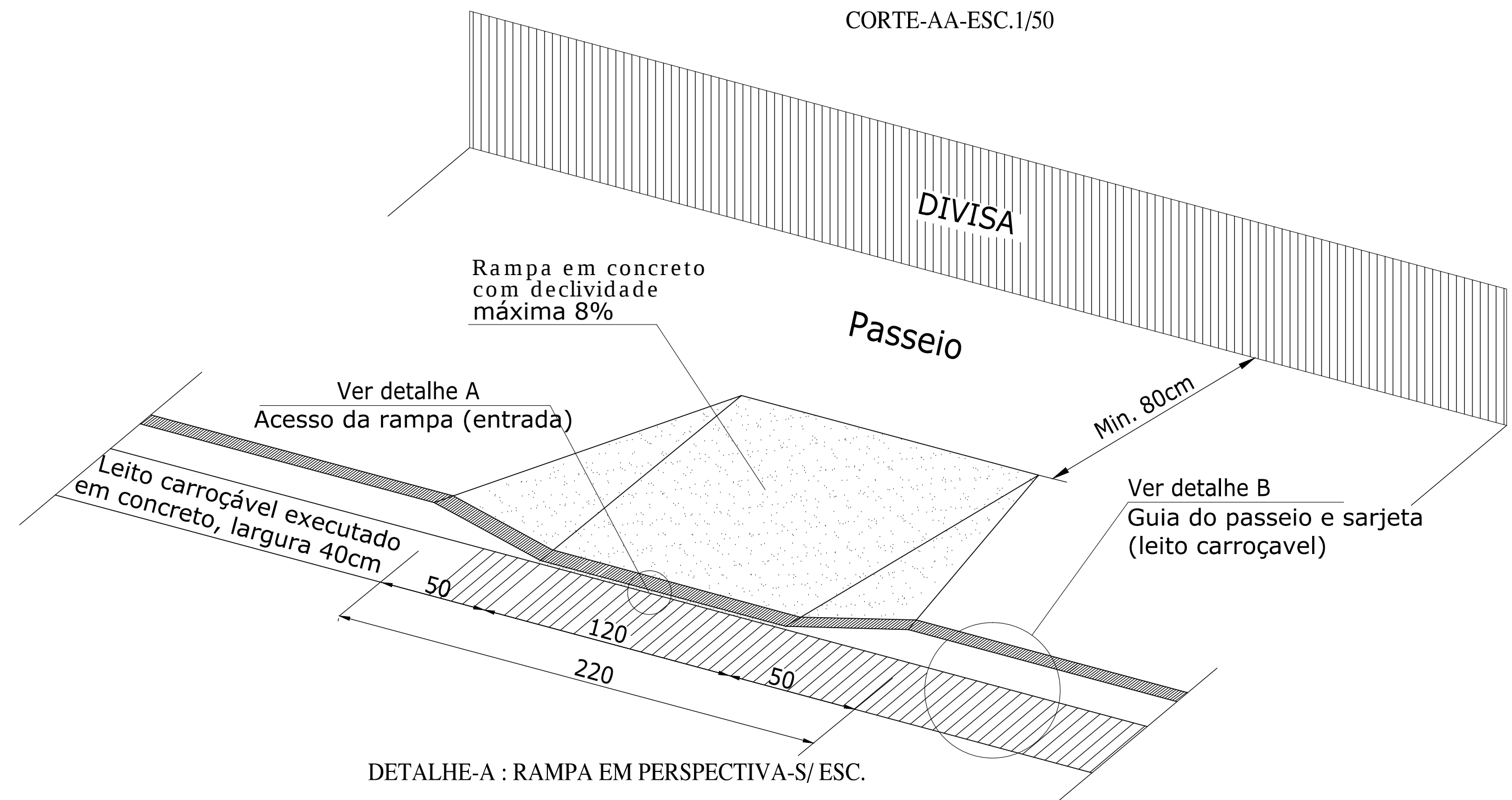
DETALHE-A : RAMPA EM PERSPECTIVA-S/ ESC.
