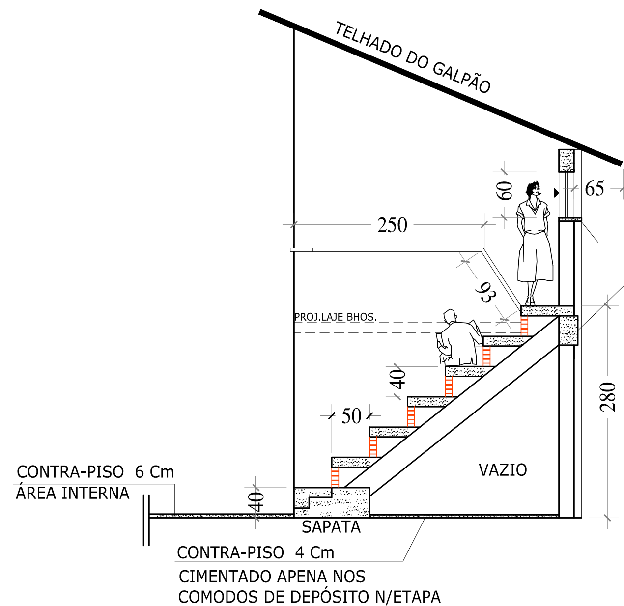
DETALHE DA ARQUIBANCADA EM CORTE-ESC.1/50 CORTE-CC
