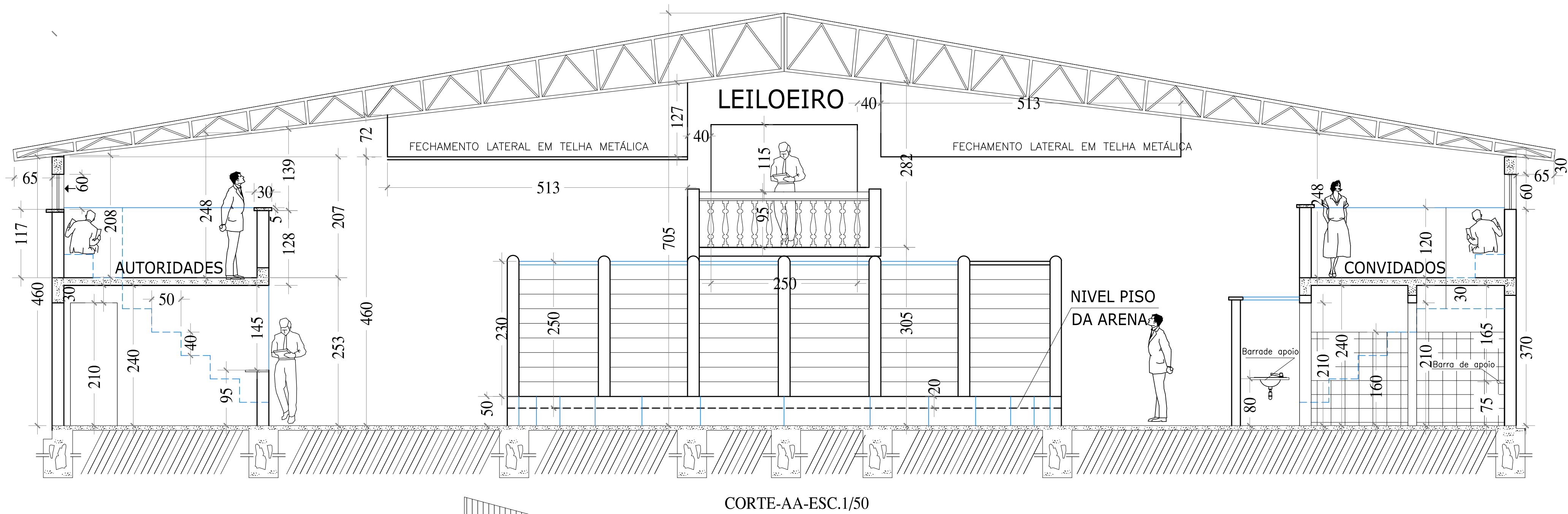
CORTE-AA-ESC.1/50
