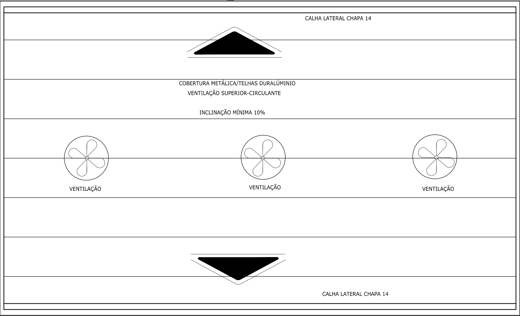
DIAGRAMA DA COBERTURA DO GALPÃO-ESC.1/100
