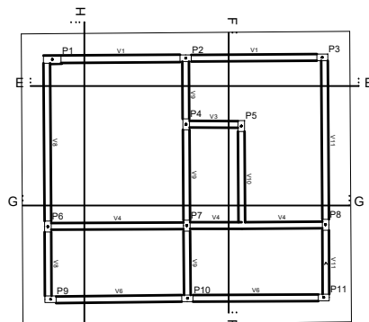
LOCALIZAÇÃO DAS LINHAS DE CORTE ESTRUTURAL-ESC. 1/50
