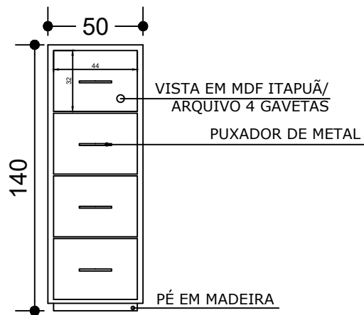
ELEVAÇÃO VISTA 2- COM MEDIDAS
