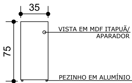
ELEVAÇÃO VISTA 1- COM MEDIDAS
