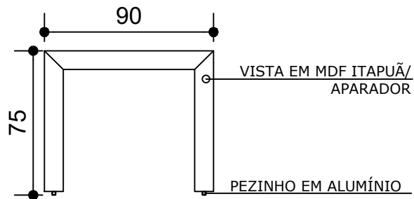
ELEVAÇÃO VISTA 2- COM MEDIDAS
