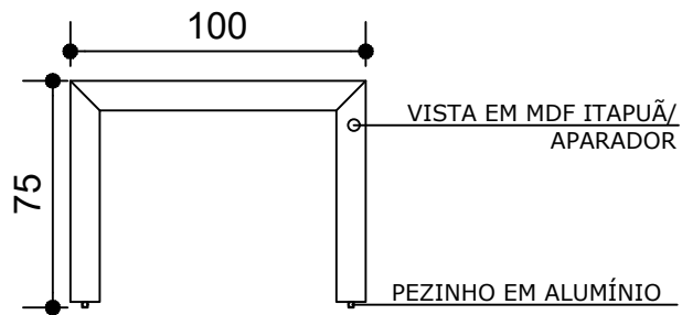
ELEVAÇÃO VISTA 2- COM MEDIDAS
