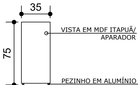
ELEVAÇÃO VISTA 1- COM MEDIDAS
