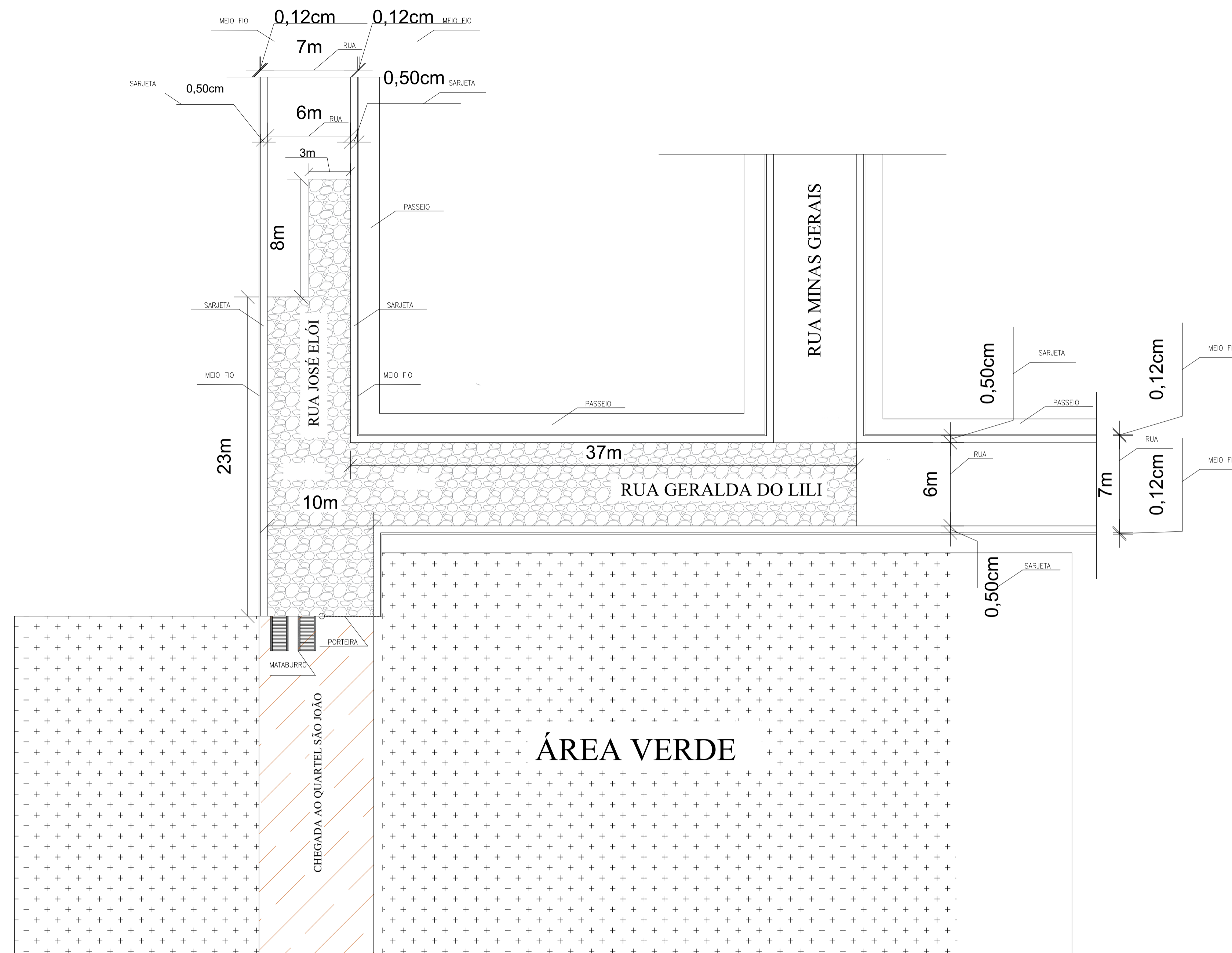
PLANTA BAIXA/PAVIMENTAÇÃO POLIÉDRICA ESC: 1/2 RUAS: JOSÉ ELÓI; RUA GERALDA DO LILI
