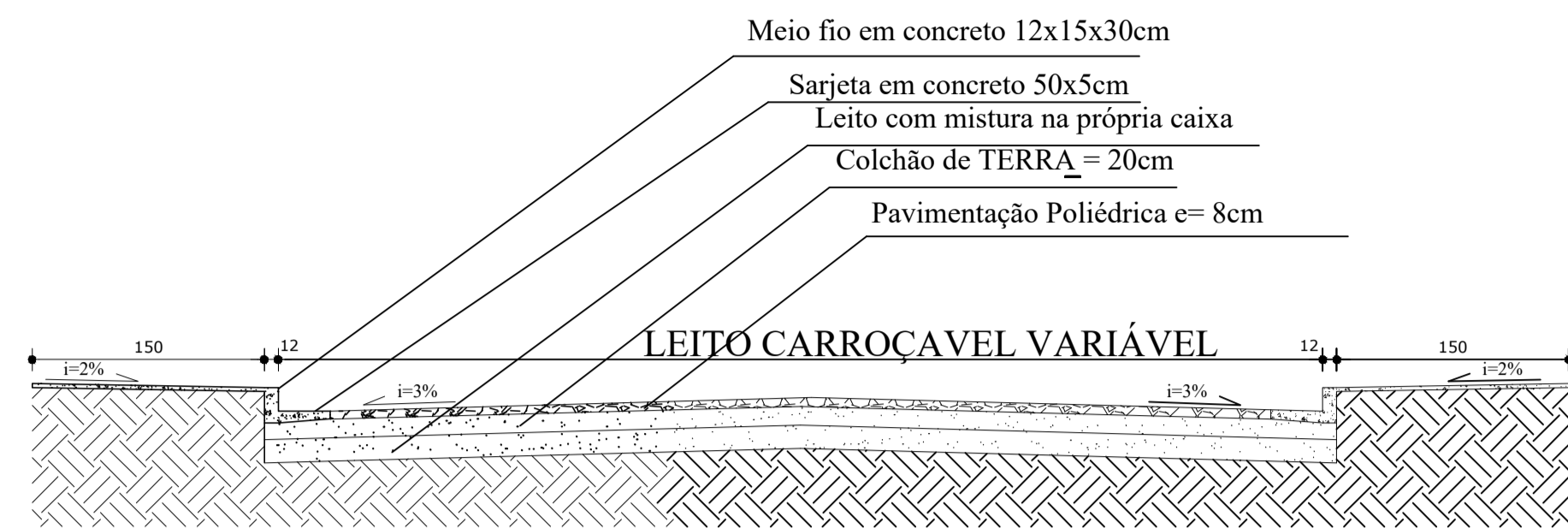
SEÇÃO TIPO (CORTE TRANSVERSAL RUAS) ESC: 1/10
