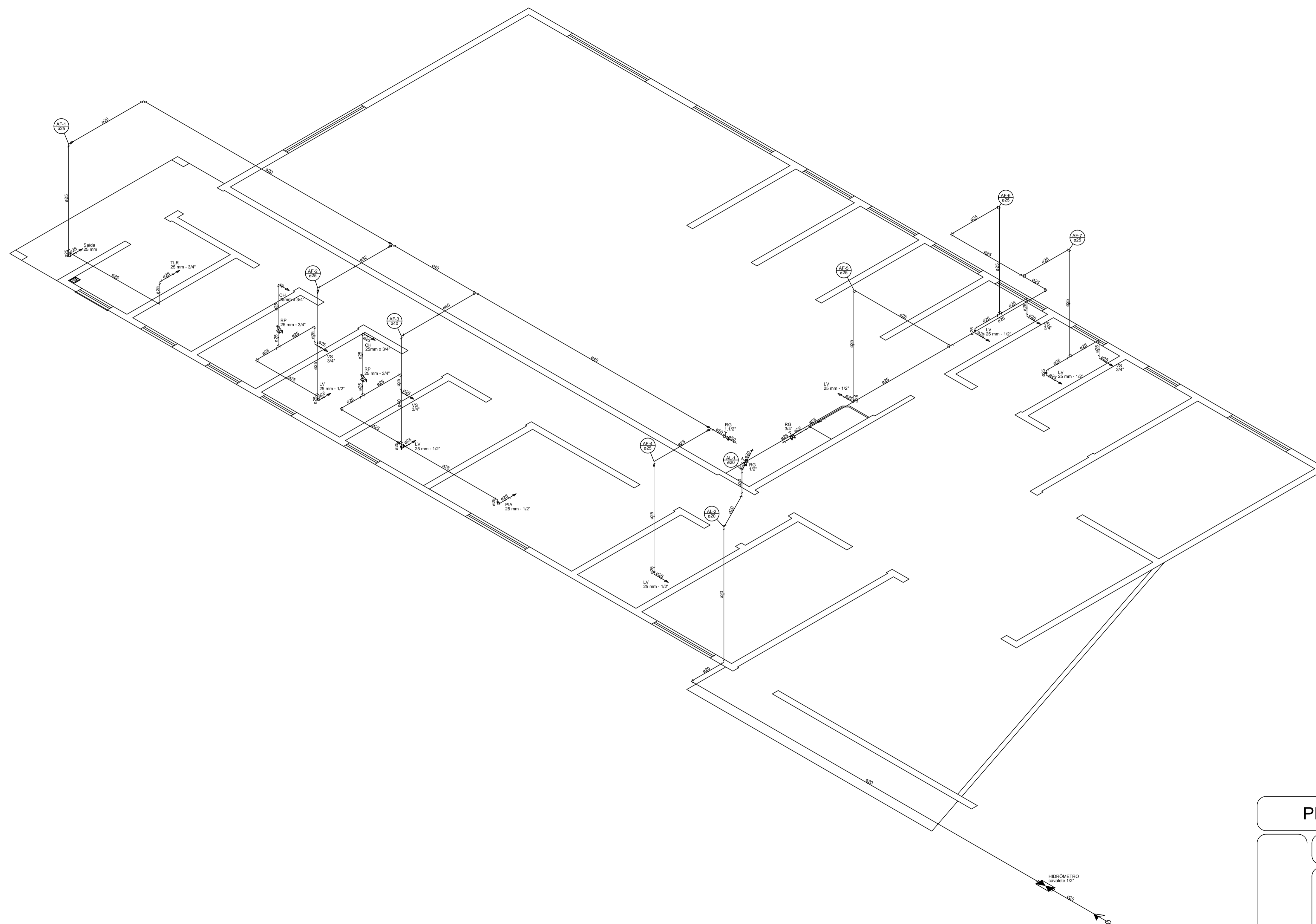
Detalhe Hidráulico Isométrico escala 1:25
