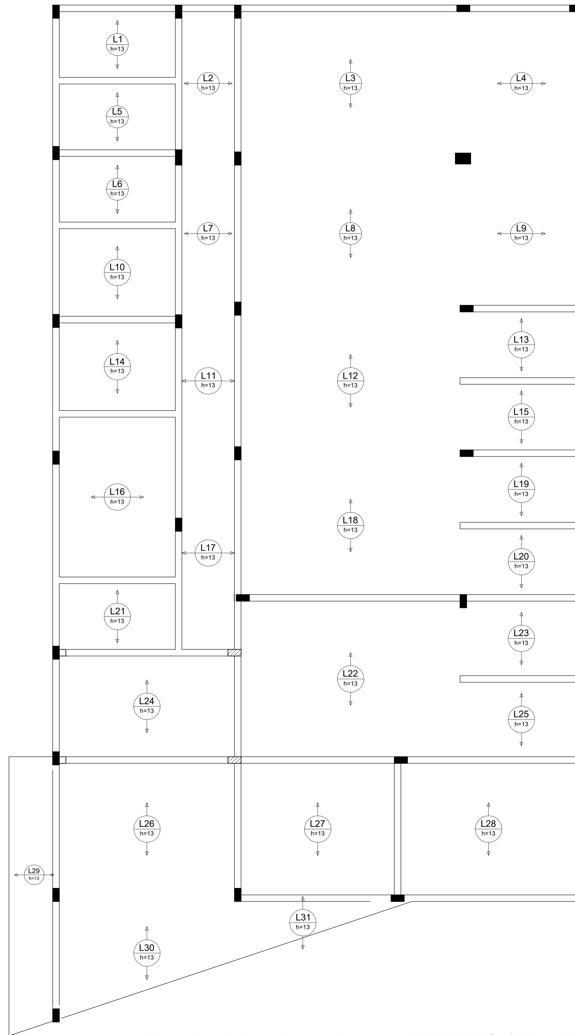
Armação positiva das lajes do pavimento TERREO (Eixo X)
