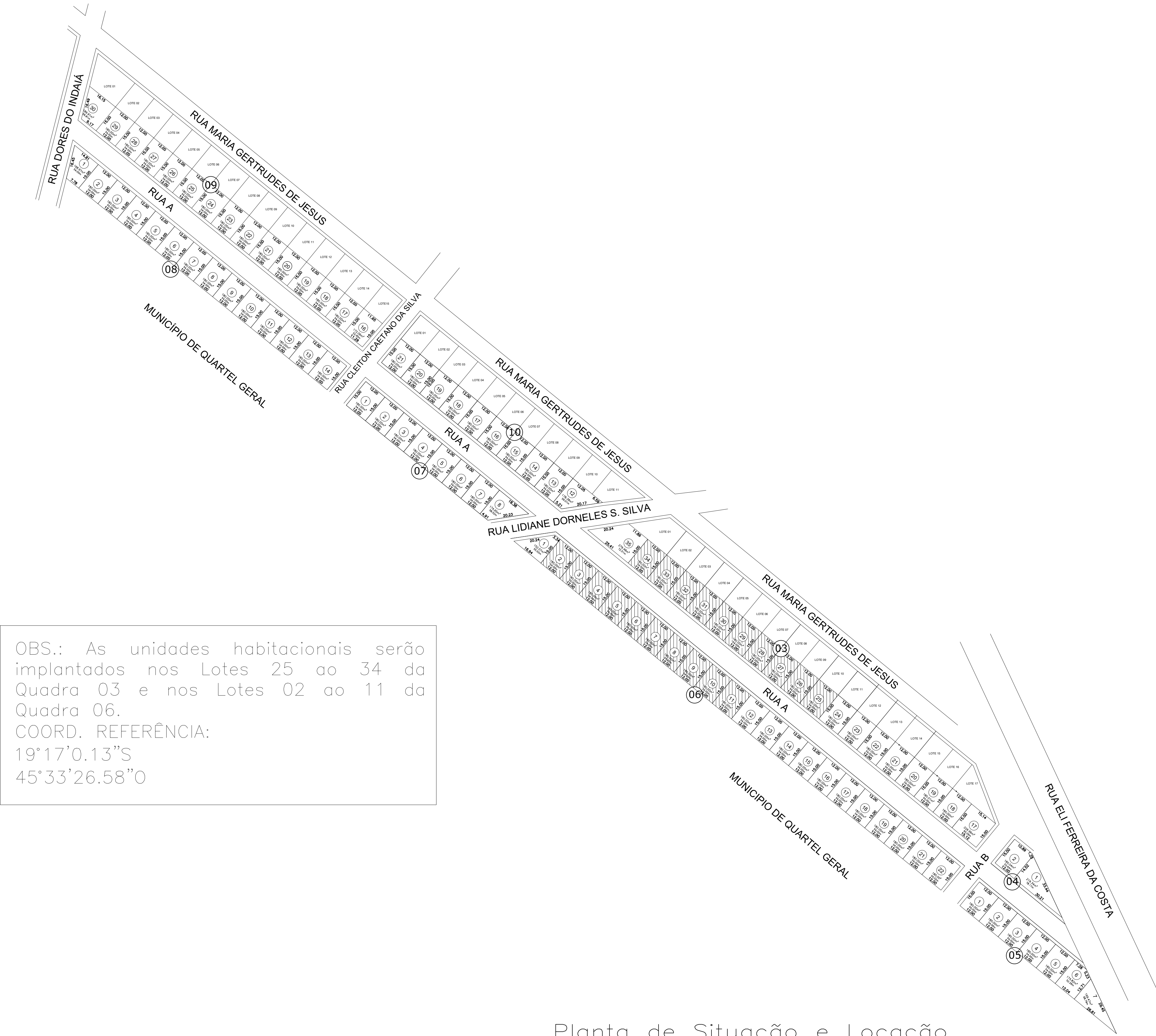
Planta de Situação e Localização ESCALA 1/1000
