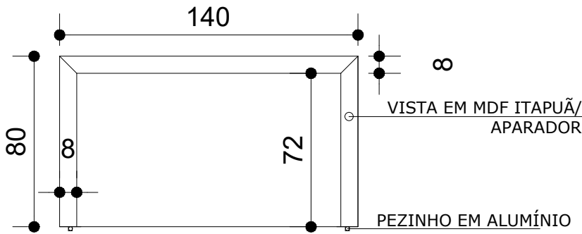
ELEVAÇÃO VISTA 2- COM MEDIDAS
