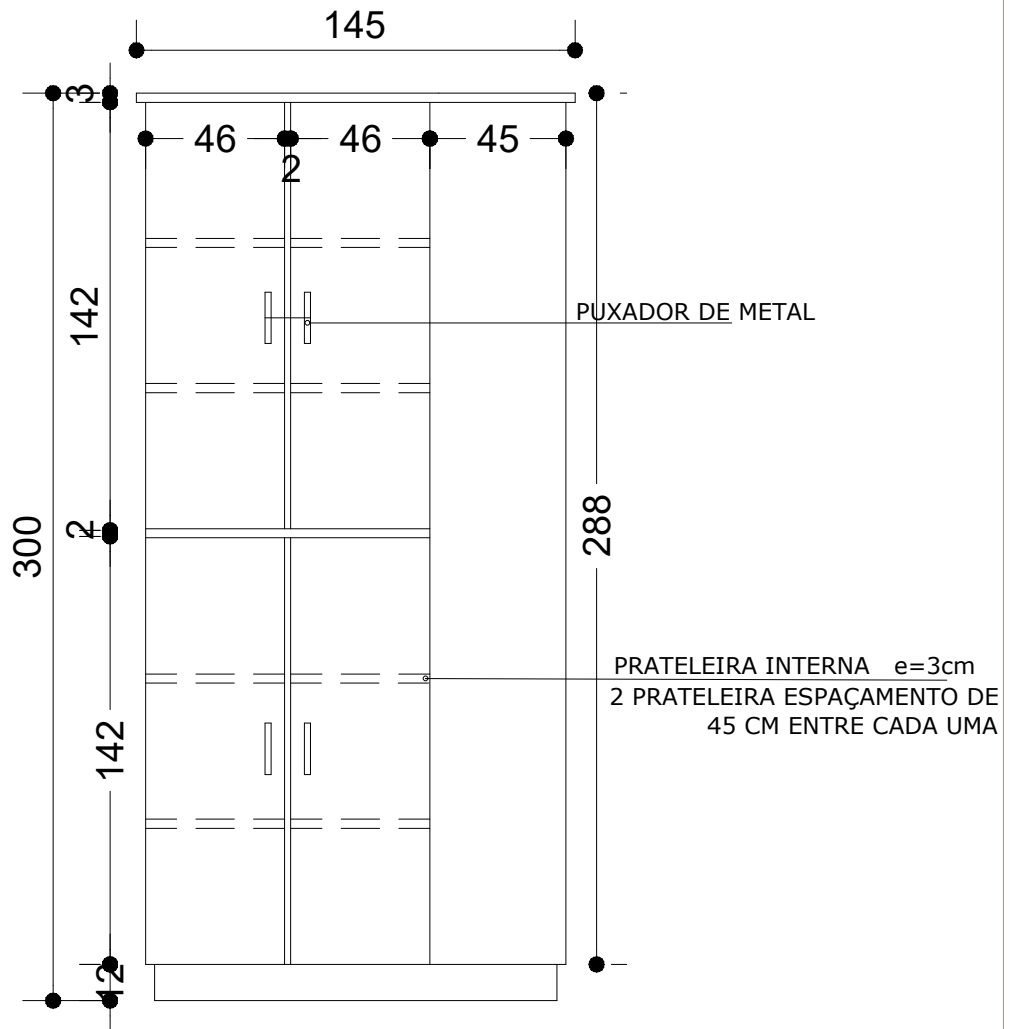
ELEVAÇÃO VISTA 3 - COM MEDIDAS
