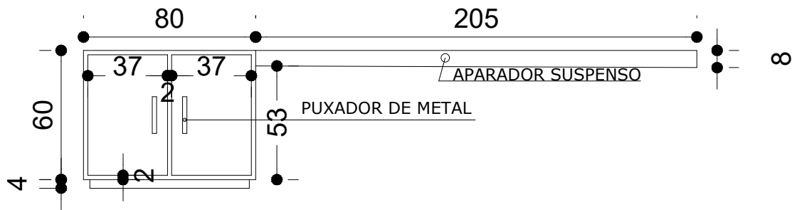
ELEVAÇÃO VISTA 2- COM MEDIDAS
