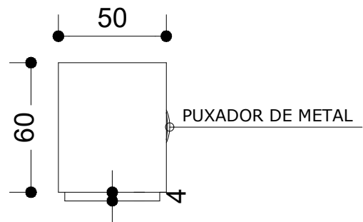
ELEVAÇÃO VISTA 1- COM MEDIDAS
