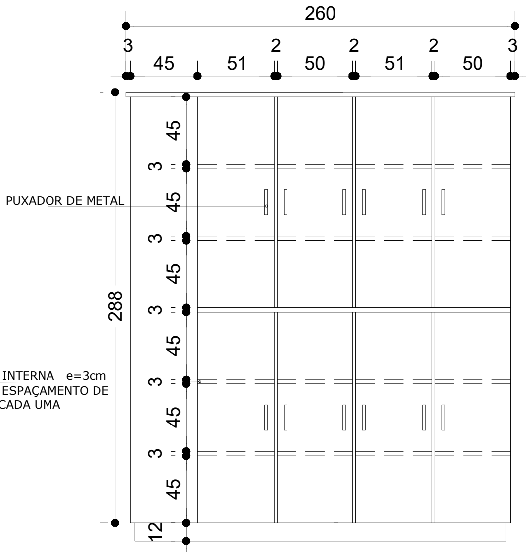
ELEVAÇÃO VISTA 2- COM MEDIDAS
