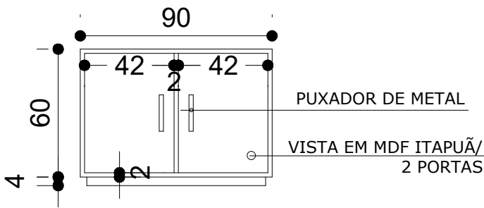
ELEVAÇÃO VISTA 2- COM MEDIDAS
