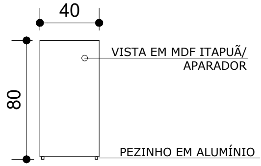
ELEVAÇÃO VISTA 1- COM MEDIDAS
