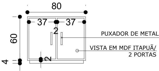
ELEVAÇÃO VISTA 2- COM MEDIDAS
