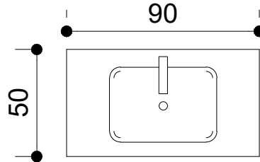
VISTA SUPERIOR COM MEDIDAS
