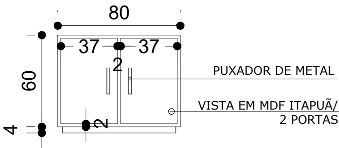
ELEVAÇÃO VISTA 2- COM MEDIDAS
